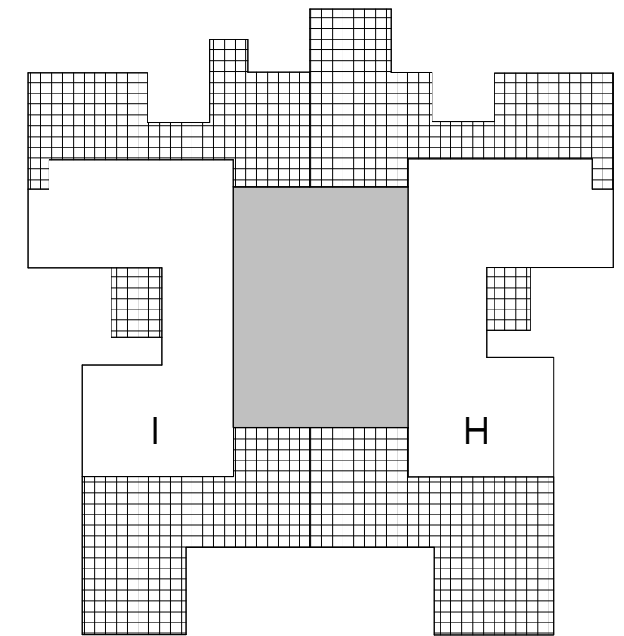
קומה 15 פנטהאוס
